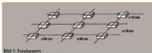
Bild 1: Fundament
