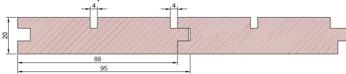
Täfer Sichtnut/Mittelnut
