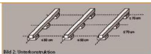
Bild 2: Unterkonstruktion
