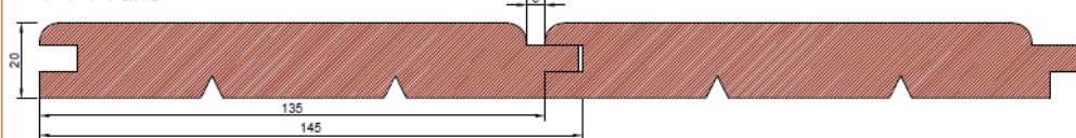
Täfer rund
