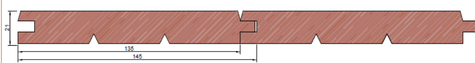
Täfer Steilfase
